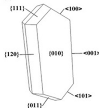
شکل ۱: بلور کامل گچ و صفحات بلوری آن (Wen-Yi Shih et al., 2005, p. 257)
