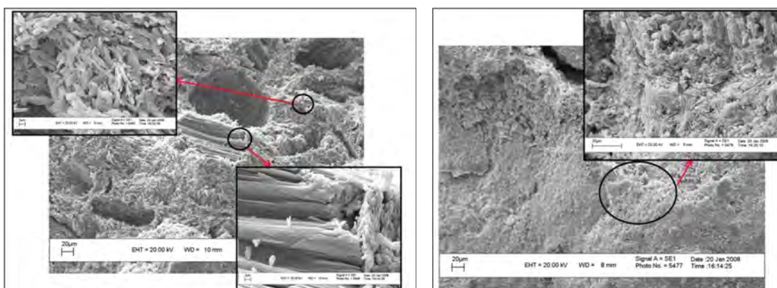
شکل ۱۱: ریز ساختار ملات گچی قلعه الموت، بزرگنمایی تصویر اصلی ۵۰۰ برابر و جزئیات ۵۰۰۰ برابر است.
