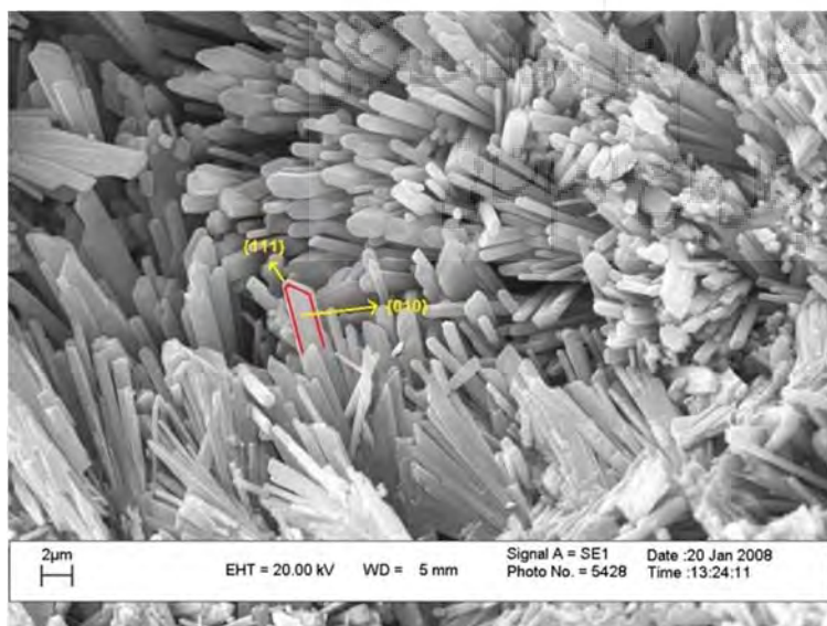
شکل ۲: تصویر SEM از گچ تیز، صفحات بلوری \{010\} و \{111\} روی یک بلور نشان داده شده است. بزرگنمایی ۵۰۰۰ برابر
