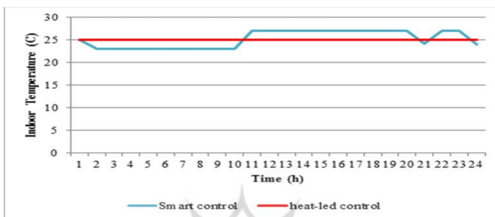
شکل ۹) دمای داخل ساختمان برای راهبردهای کنترلی heat-led و هوشمند
