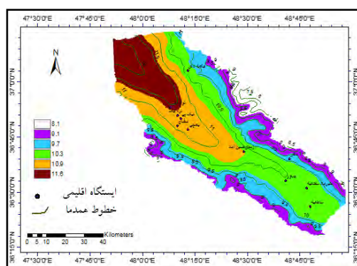
شکل (۶) خطوط همدمای حوضه زنجان رود
