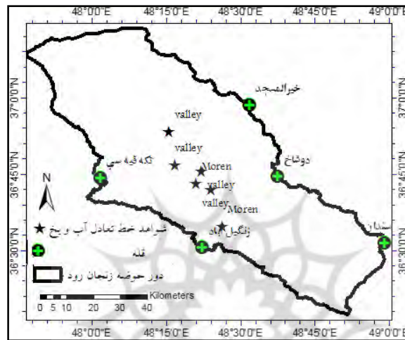
شکل (۱۰) بلندترین قله‌های منطقه و شواهد خط تعادل آب و یخ مجاور آن‌ها
