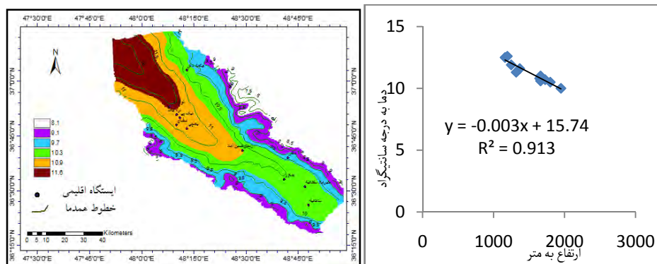
شکل (۵) رابطه بین دما با ارتفاع
