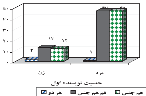
نمودار ۸. جنسیت همکاران بر حسب جنسیت نویسندگان اول در مقالات مشترک
